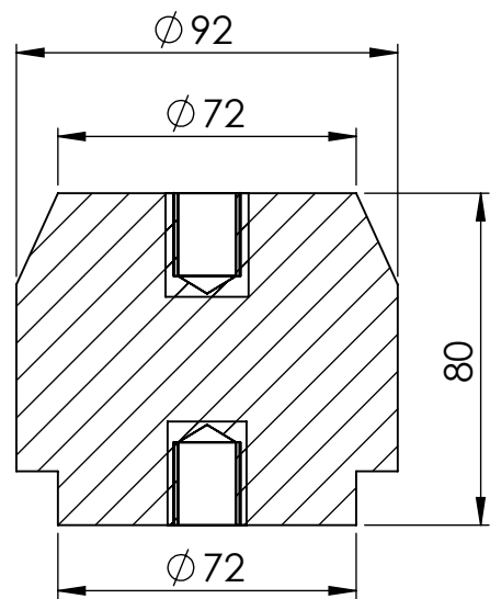
SEÇÃO A-A
