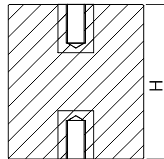
SEÇÃO A-A
